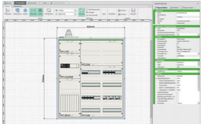
Konfiguration eines Verteilers
