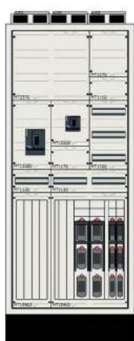
Modulansicht offen
