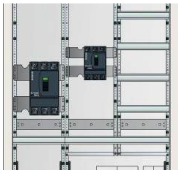
Modulansicht offen
