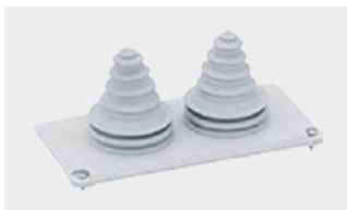
GKT26 Leitungseinführungsplatte, für M, S, SV, SF, SP, SE-Gehäuse, mit Kabelstutzen, für Kabel 2 x 14 – 54 mm
