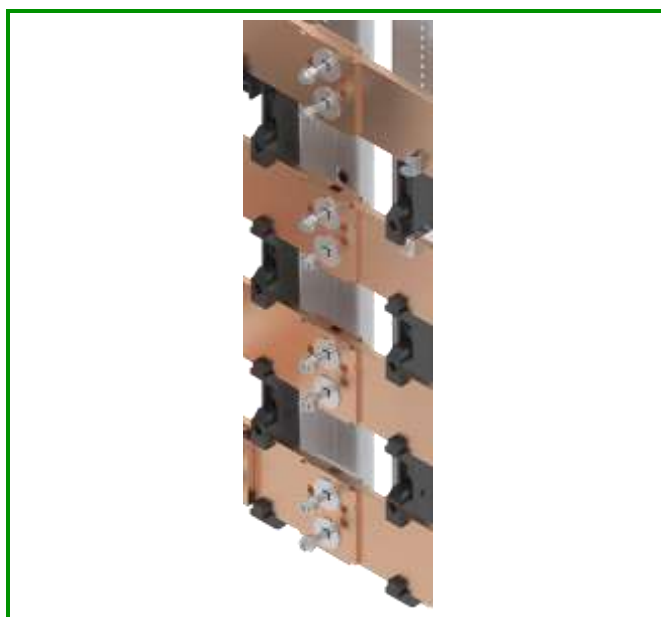
Unten: 4 x waagrechte Schrank-Schrank-Verbindung LVS04641 (1600 A) für N, L1, L2 und L3
