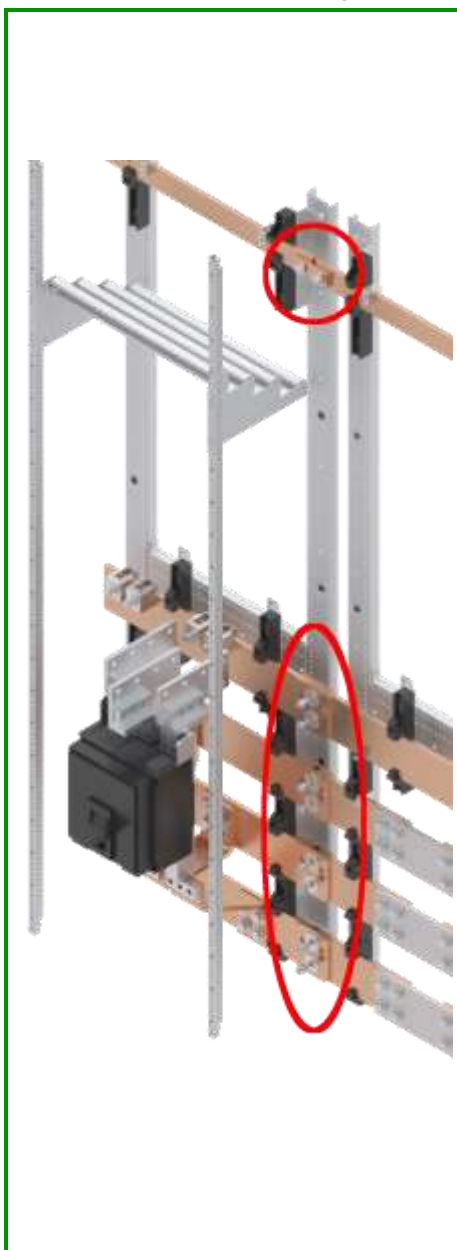
Oben: Waagrechte Schrank-Schrank-Verbindung XSV1213 für PE
