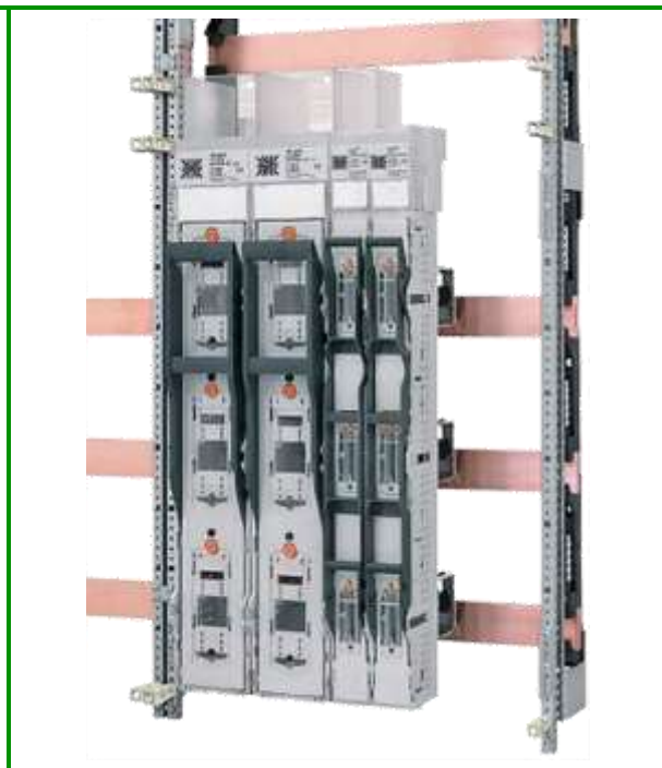
Systemlösung 185 mm Sammelschiene für Sicherungsbehaltete Einbaugeräte (NH00, NH1, NH2, NH3)
