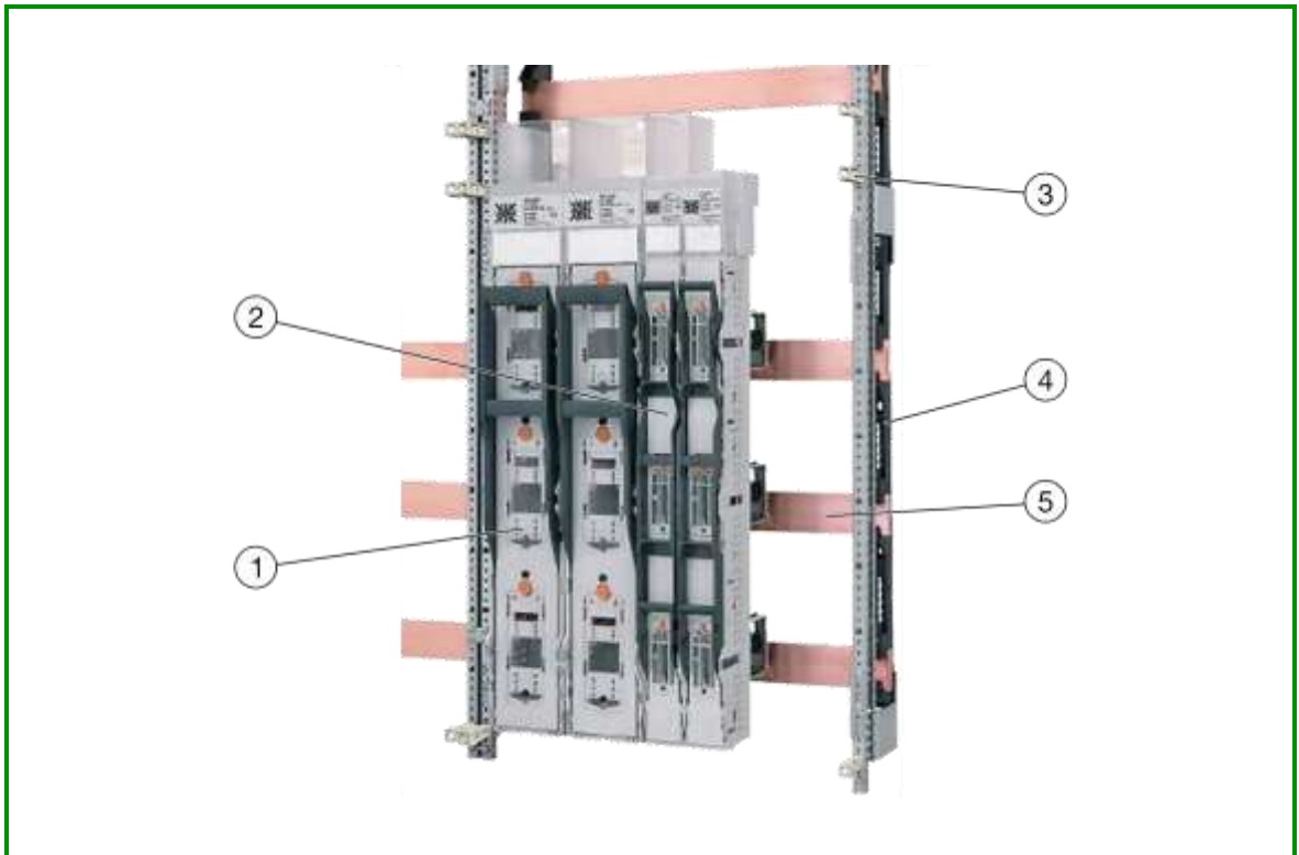
185 mm und 100 mm Sammelschienensystem - Systemübersicht mit Beispielergeräten (hier je 2 x NH-Sicherungslastschaltleiste XTL9x2W und XTL903)
